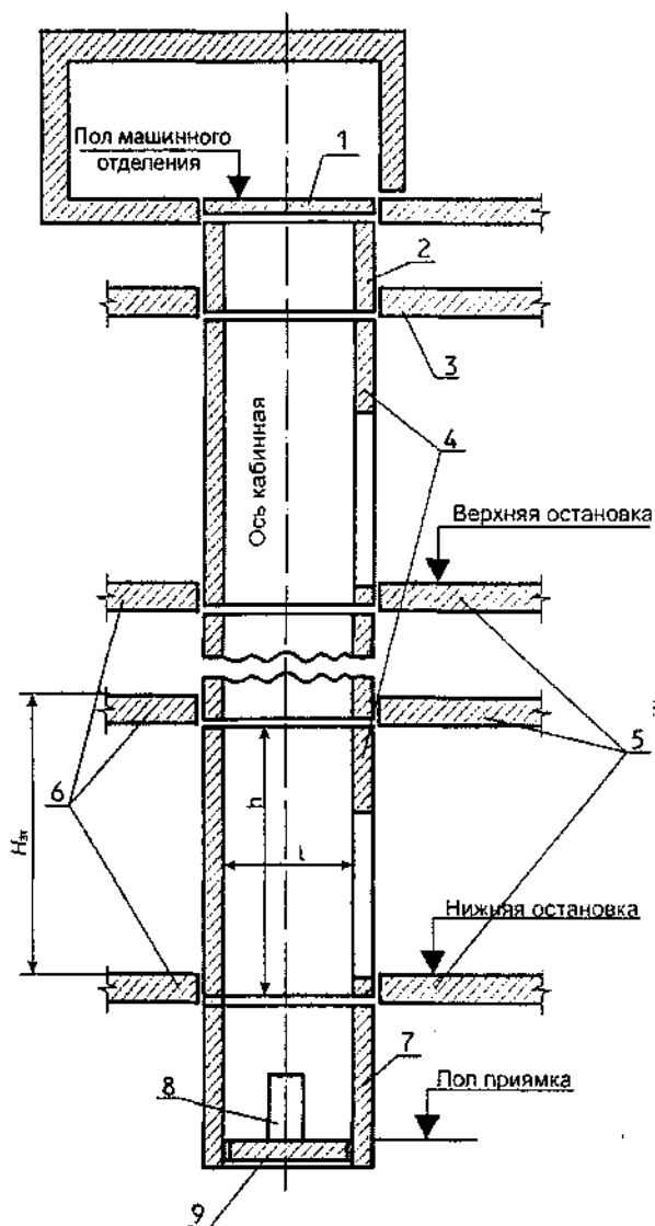
Схема шахты лифта
