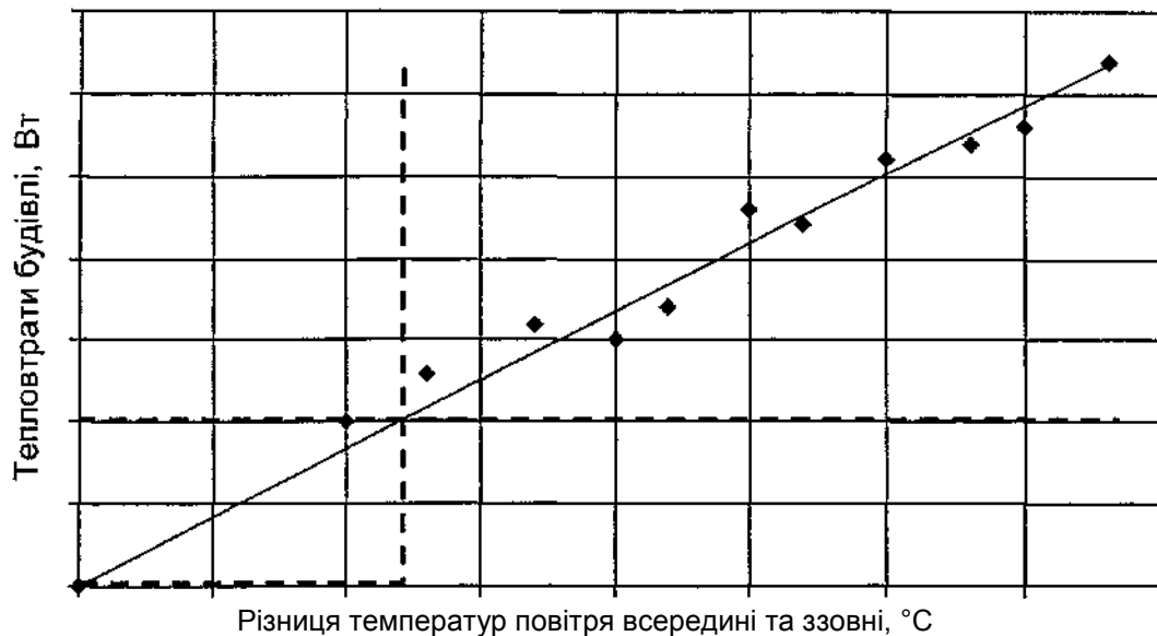
Рисунок 1 - Схема функціональної залежності тепловтрат будівлі від різниці температур повітря всередині та ззовні
