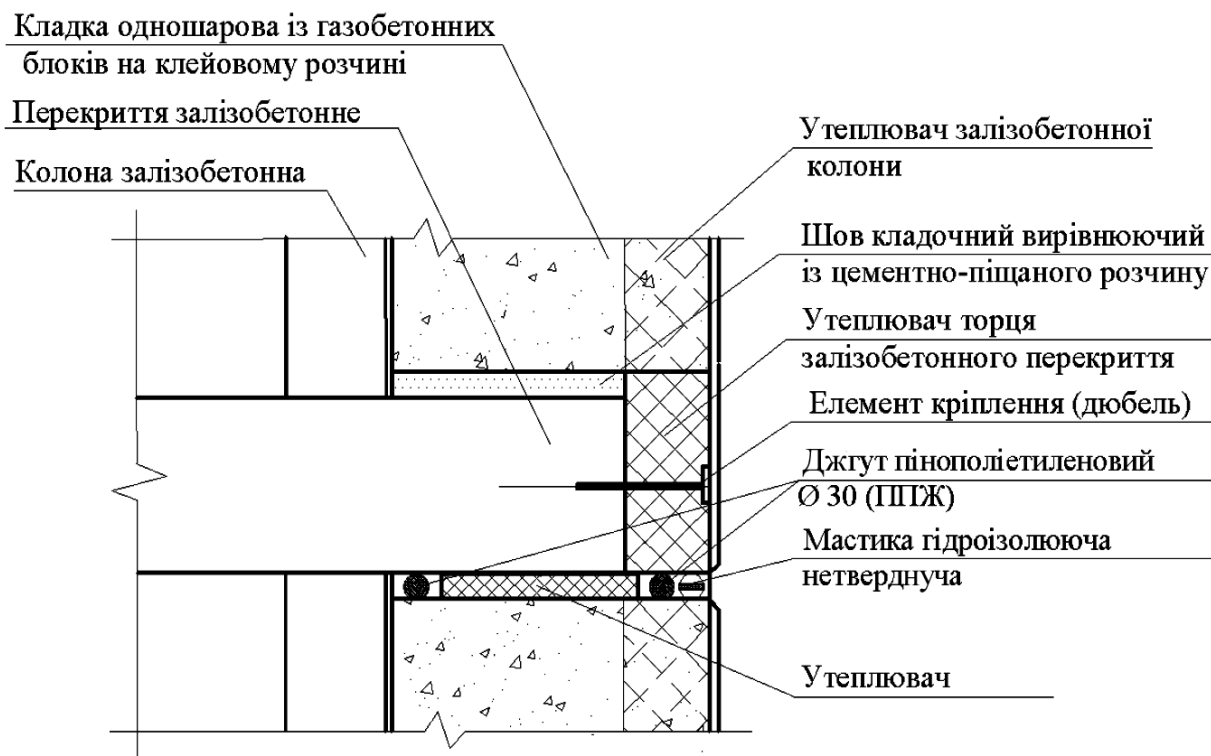
Рисунок 6.1 – Конструктивне рішення влаштування вузла примикання стіни із газобетонних блоків до перекриття
