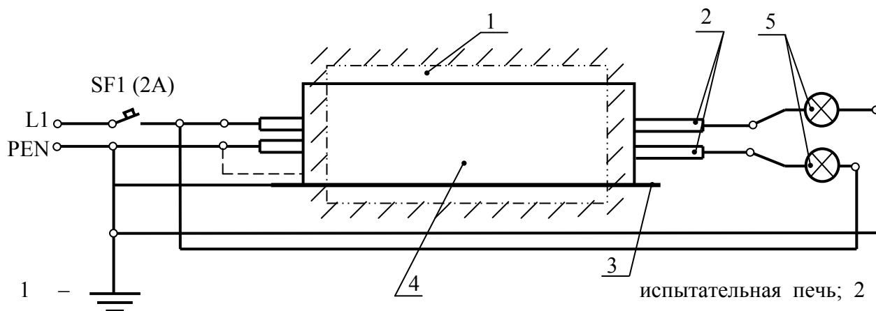
1 – испытательная печь; 2 – кабельная линия; 3 – элементы крепления образца в печи; 4 – кабельный короб; 5 – электролампы накаливания; L1– источник однофазного напряжения; PEN – заземленный нейтральный проводник; SF1 (2A) – выключатель или предохранитель
