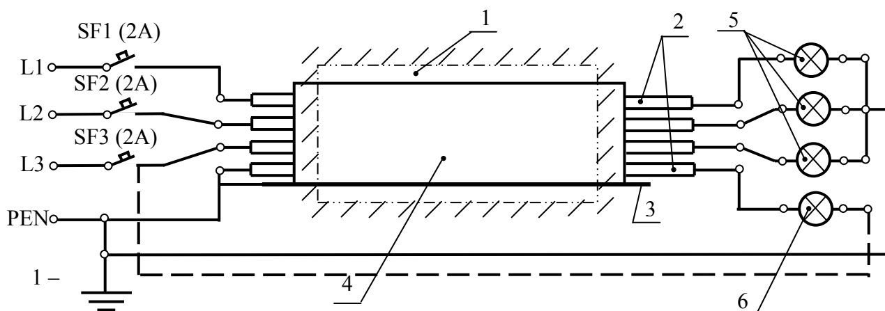
испытательная печь; 2 – кабельная линия; 3 – элементы крепления образца в печи; 4 – кабельный короб; 5 – электролампы накаливания; L1, L2, L3 – источник трехфазного напряжения; PE – заземленный нейтральный проводник; SF1-SF3 (2A) - выключатели или предохранители; 6 – электролампа накаливания в сети нейтрального проводника.
